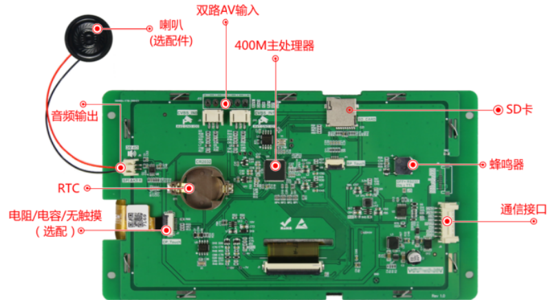
图 1-4 硬件配置图
